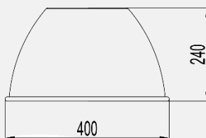
Chóa đèn 120°
